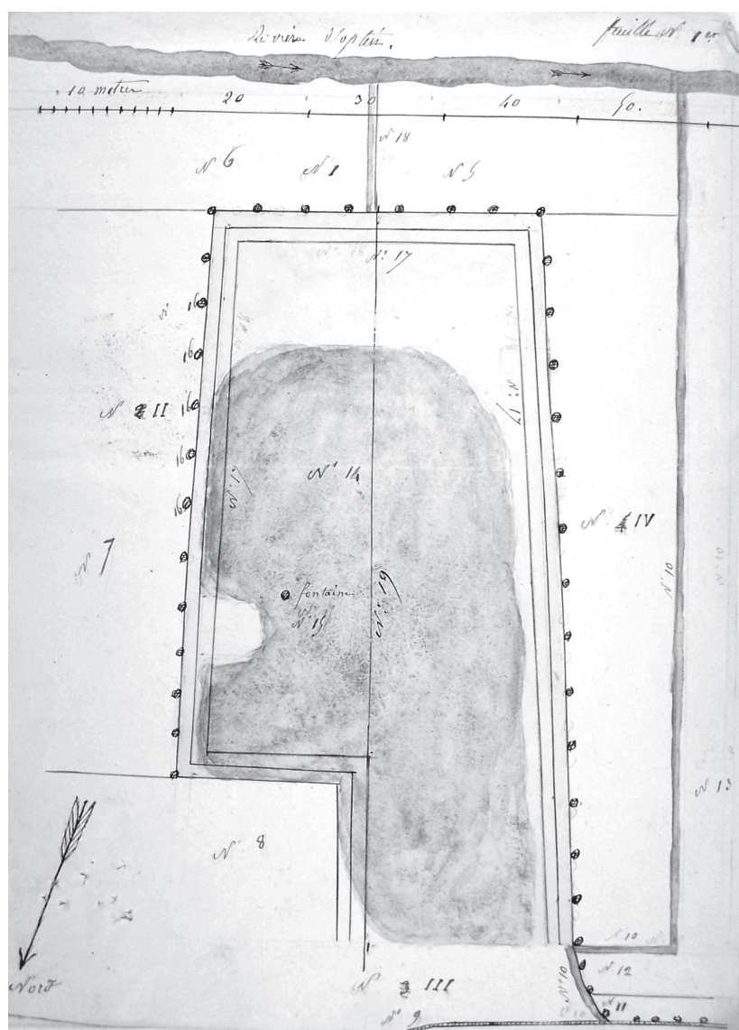
BOUCHY-LE-REPOS, plan du lavoir projeté en 1842, avec fontaine à l'intérieur, et délimitation, Arch. Marne, 2 O 604
