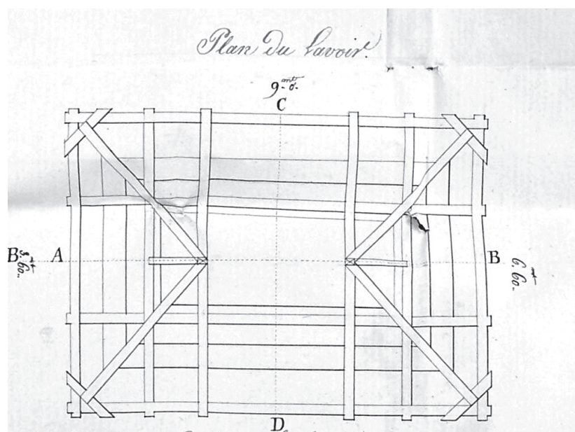
SUIZY-LE-FRANC, plan du lavoir à établir, 27 mars 1820, Arch. Marne, 2 O 4361
