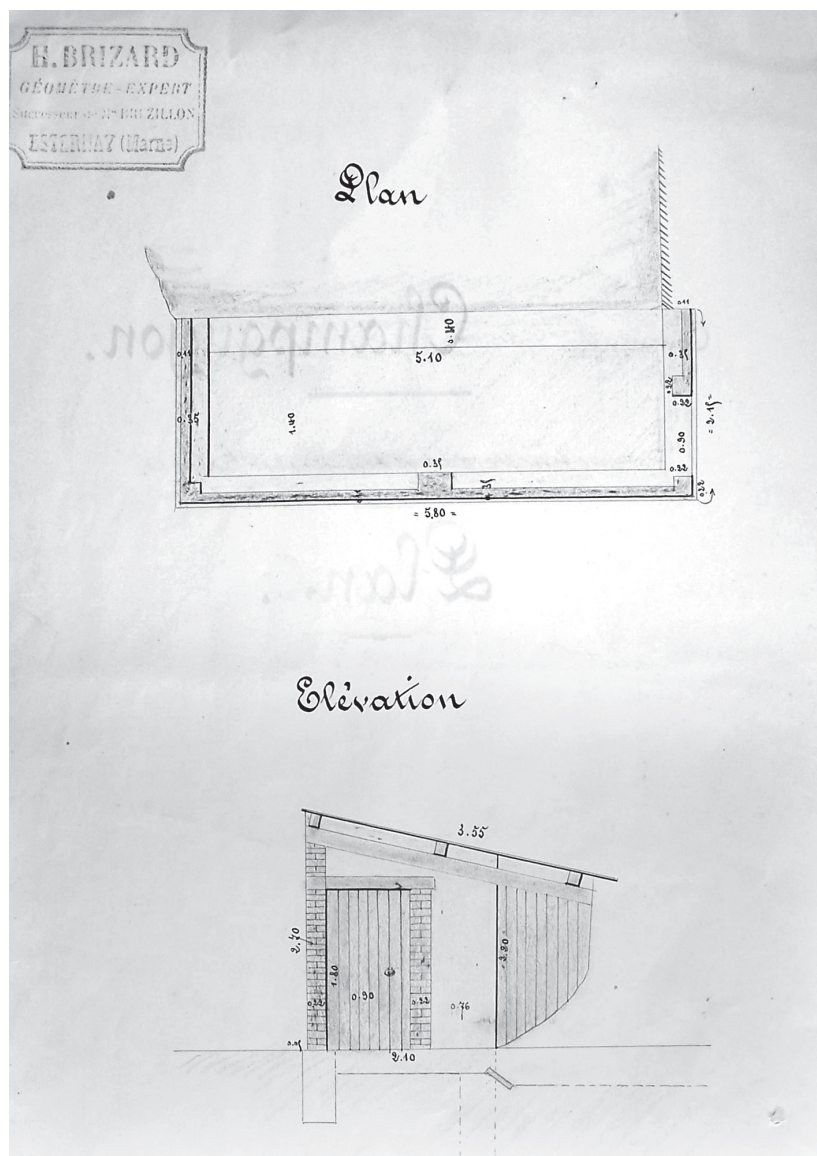
CHAMPGUYON, plan du lavoir couvert sur le Gué-du-Val, 10 novembre 1911, Arch. Marne, 2 O 982
